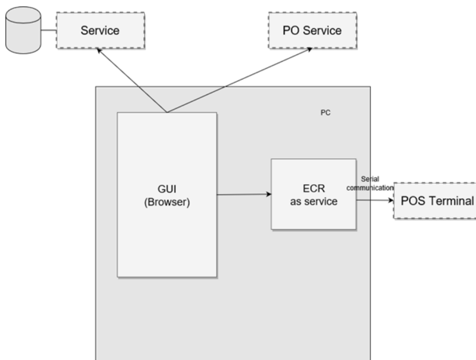
Слика 2. Поједностављена архитектура система
