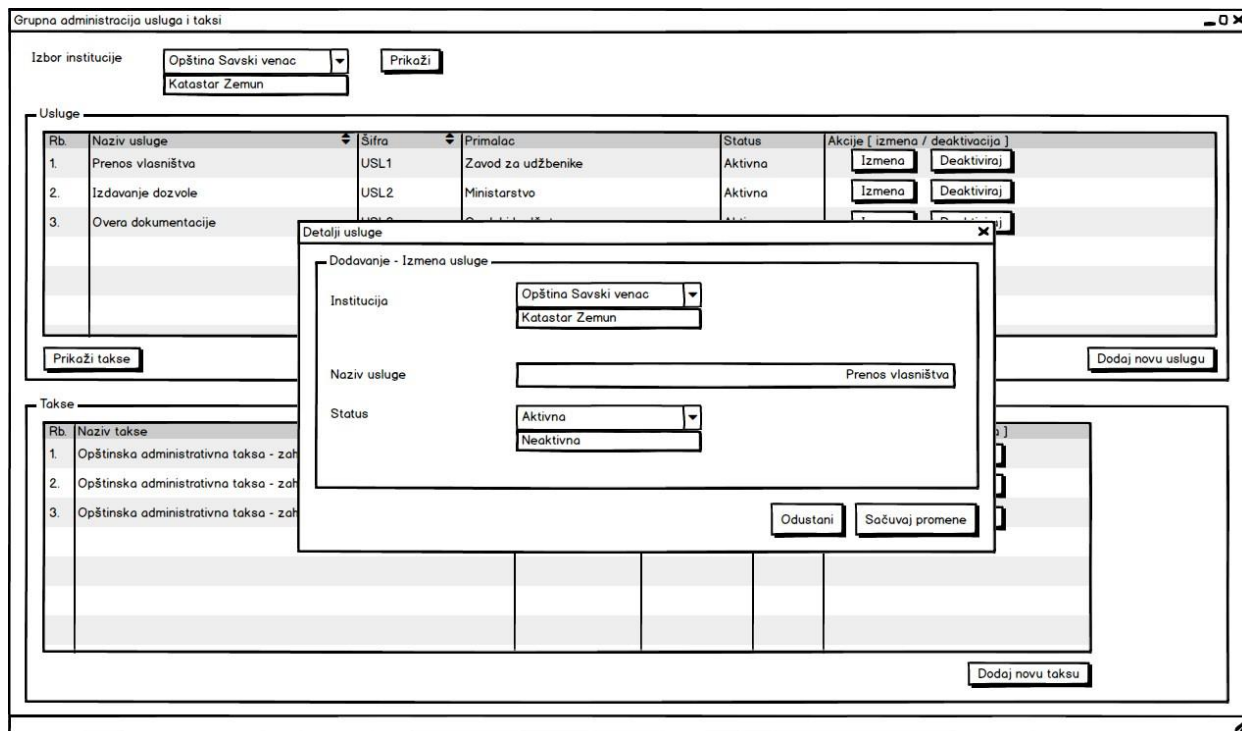
Слика 12. Предлог изгледа екрана за групну администрацију услуга – детаљи услуге
