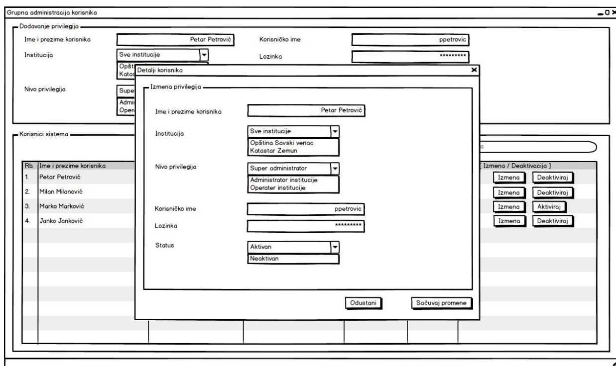
Слика 10. Предлог изгледа екрана за групну администрацију корисника – детаљан приказ корисника
