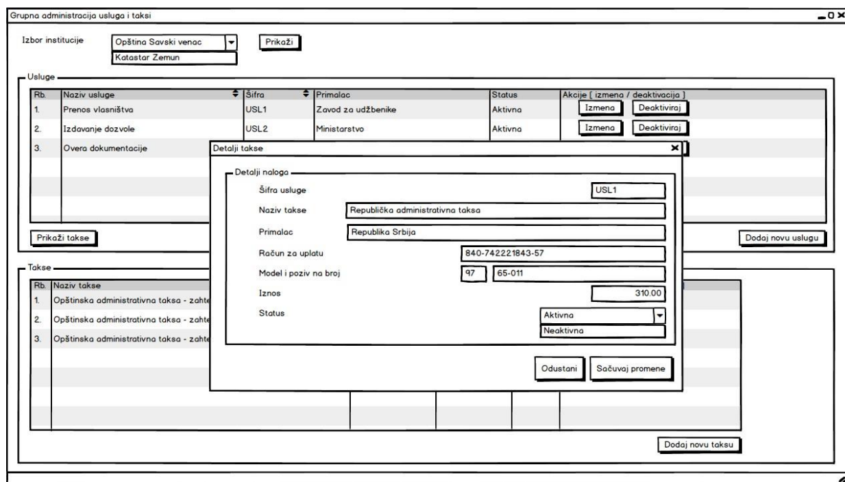
Слика 13. Предлог изгледа екрана за групну администрацију услуга – детаљи услуге
