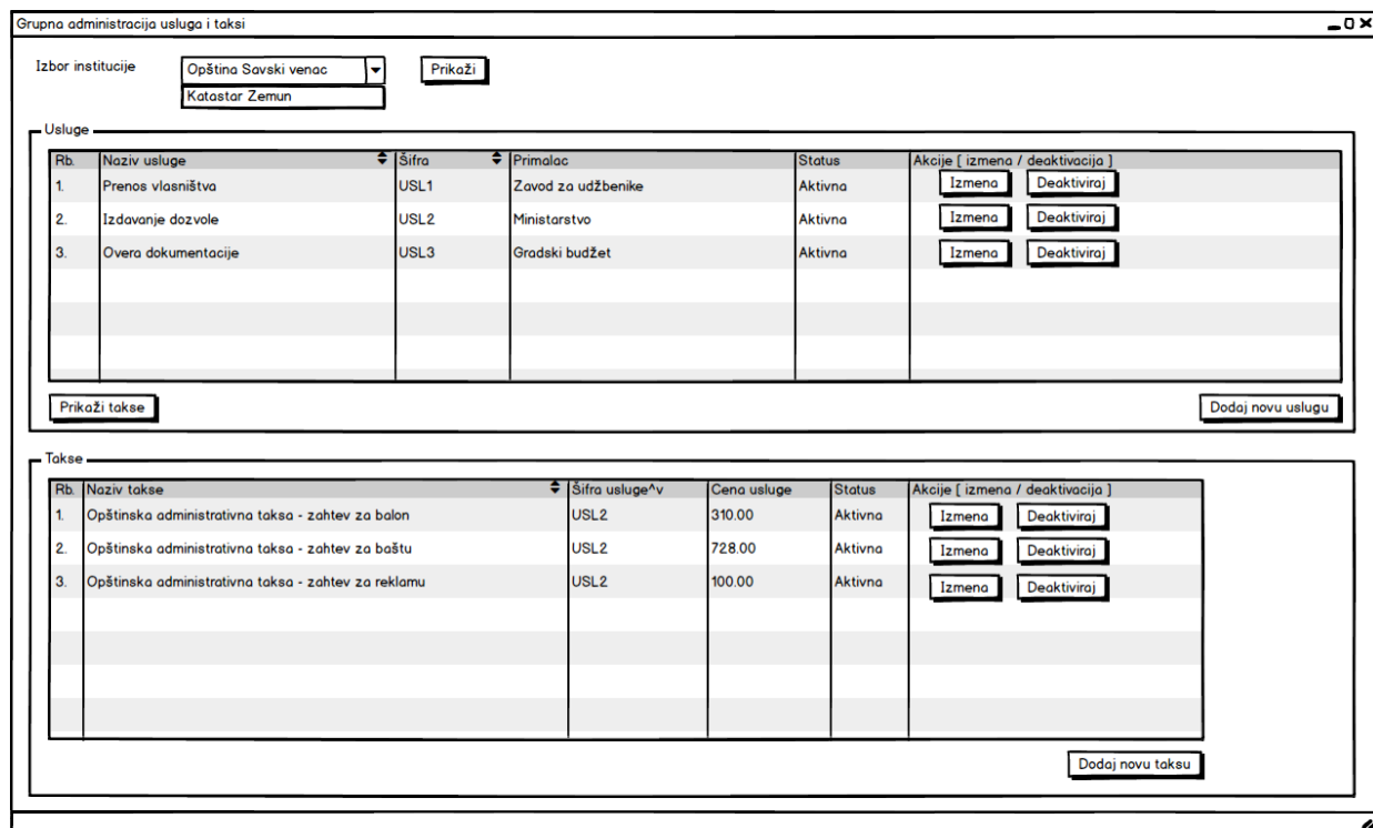
Слика 11. Предлог изгледа екрана за групну администрацију услуга
